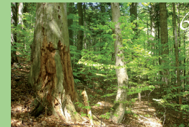
Natürlicher Mischwald
